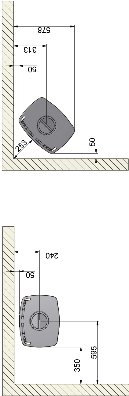
Minimale afstand tot brandbare muur (zonder zijglas)
