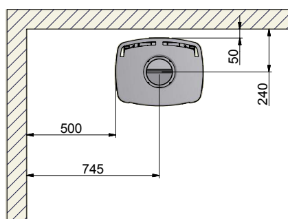
41-2 (met zijglas) Parallele installatie
