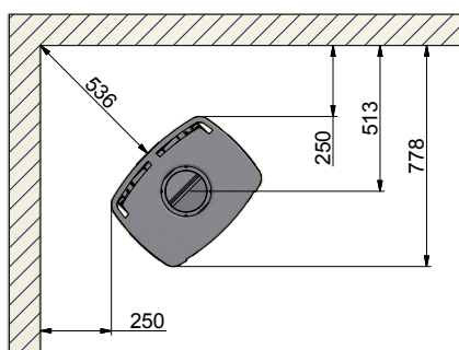
41-2 (met zijglas) Installatie in een hoek van 45°
