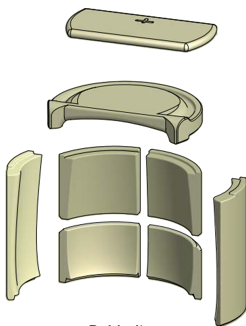
Bekleding van de verbrandingskamer
