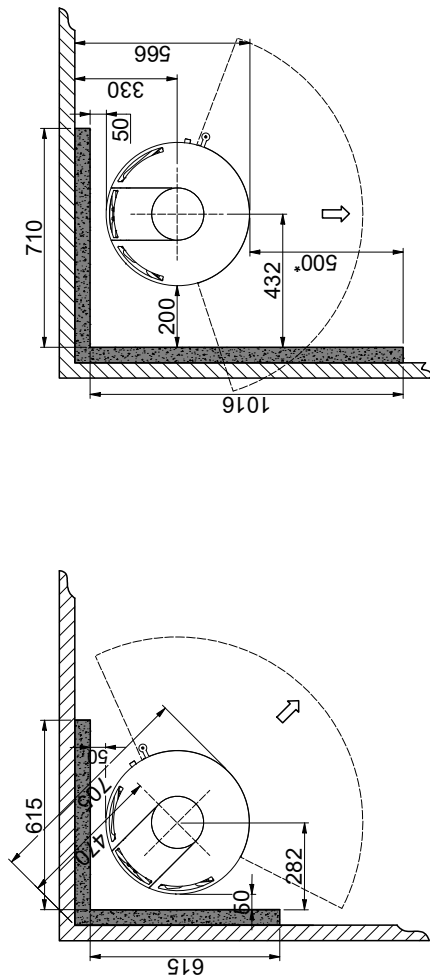
Minimale afstand tot brandbare muur beschermd door brandmuur
